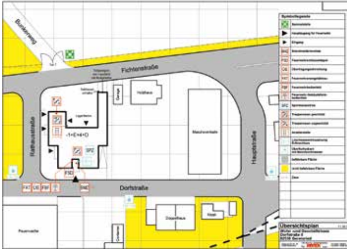
Abbildung 1: Feuerwehrplan nach DIN 14095 (hier der Übersichtsplan) (Quelle: SFSG)
