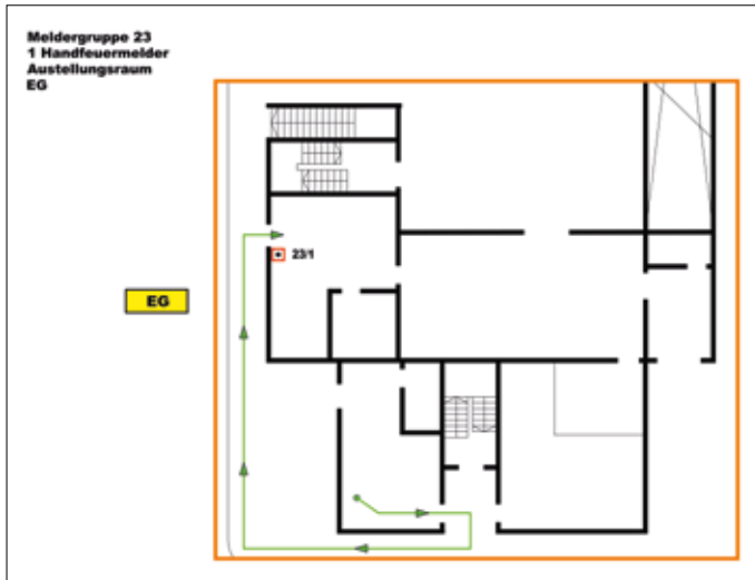
Abbildung 4: Feuerwhehraufkarte (hier die Rückseite) (Quelle: SFSG)
